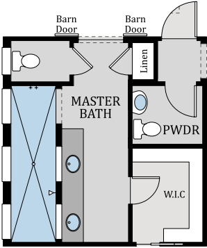
OPTIONAL 1/2 BATH ILO W.I.C.
